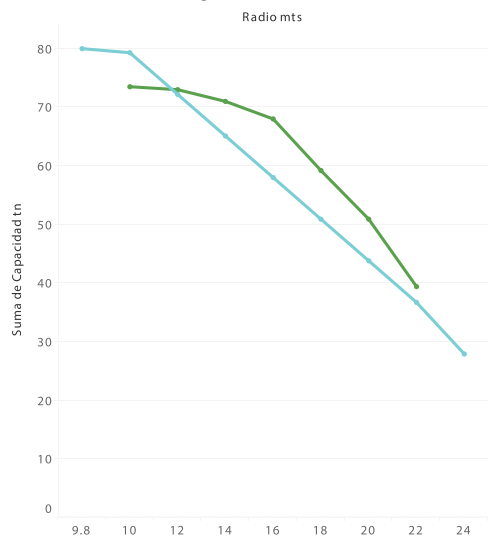
Boom 21 m + Luffi ng 21 m (88°) / tn
