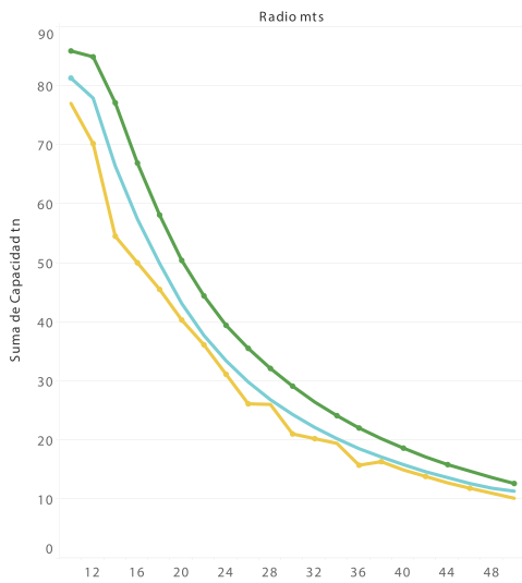
Boom 56 mts / tn
