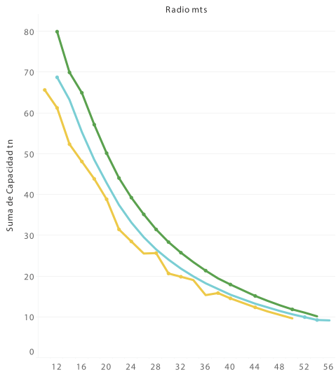
Boom 62 mts / tn
