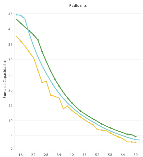
Boom 80 mts / tn
