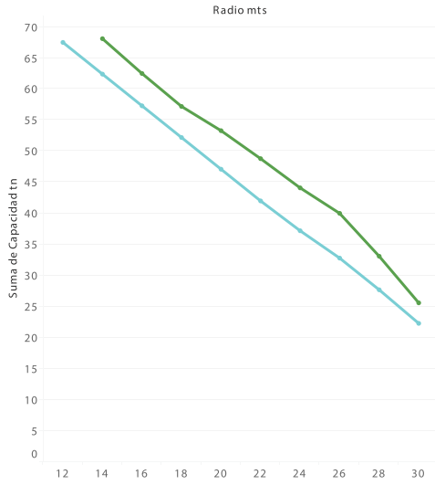
Boom 27 m + Luffi ng 27 m (88°) / tn
