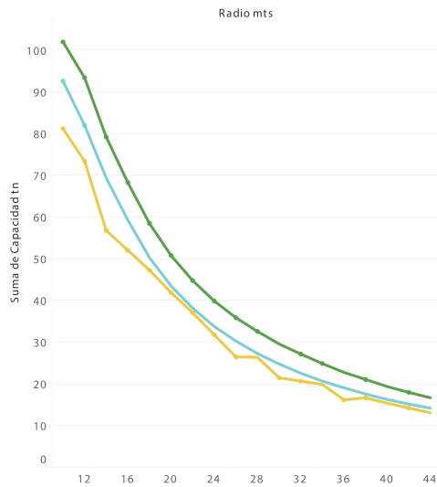
Boom 50 mts / tn
