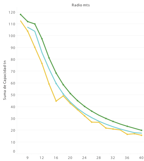
Boom 44 mts / tn
