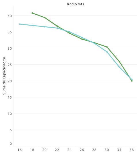
Boom 39.6 m + Luffi ng 39.6 m (85°) / tn
