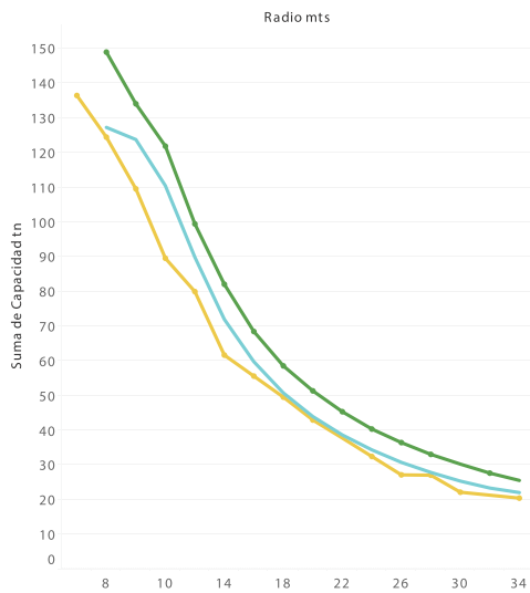
Boom 38 mts / tn
