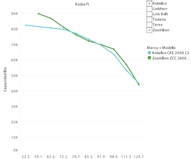
Boom 129.92 ft + Luffi ng 129.92 ft (85°) / lbs
