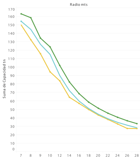
Boom 32 mts / tn
