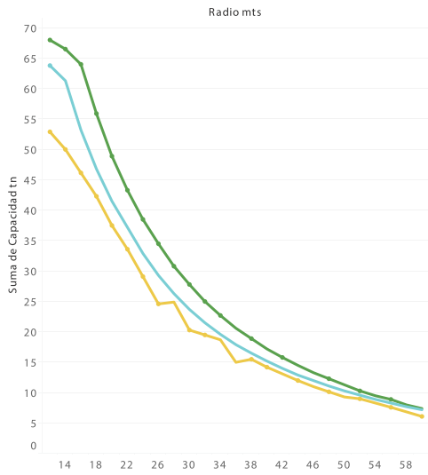
Boom 68 mts / tn
